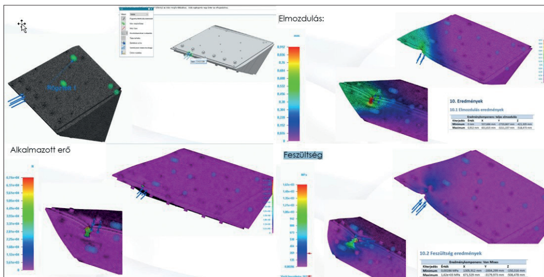
20. ábra: Leopard 2A6 frontpáncél lövedék roncsolási szimulációs részletek
