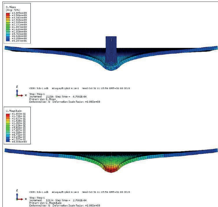
4. ábra: 3 mm-es meglőtt lemez színeképes szimulációs deformáció eredmény (Abaqus szoftver)
