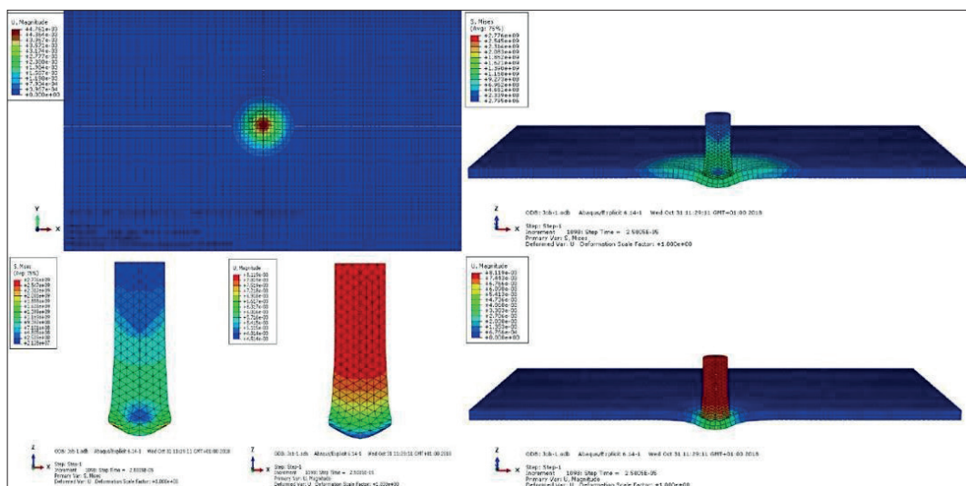
3. ábra: 4 mm-es meglőtt lemez simulációs kivonat sorozat lövedék deformációs modellel (Abaqus szoftver)
