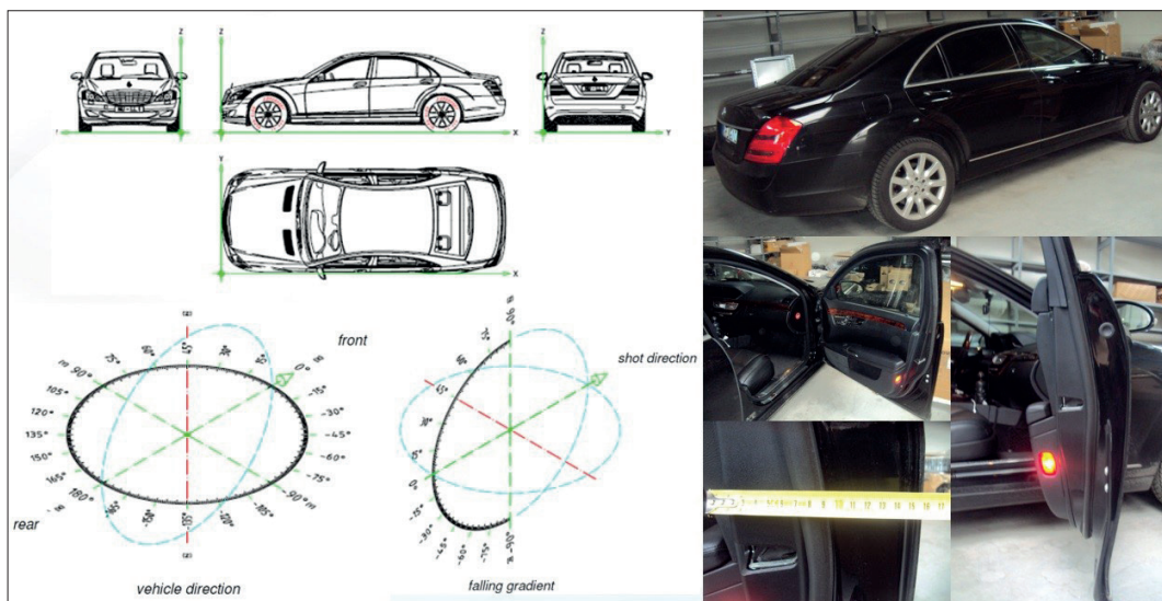
9. ábra: VPAM tesztkörnyezeti illusztráció
