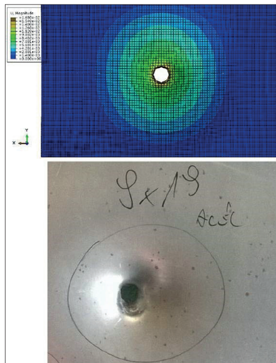
5. ábra: 2 mm-es lemez Abaqus szimuláció tesztlövés fényképével összevetése
