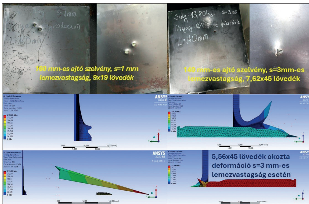
12. ábra: Meglőtt minták Ansys elemzései
