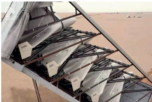
4. sz. ábra: Shahed–136 nem visszatérő (Ukraine claims to have shot down 20 Iranian-built Shahed drones during mass attack by Russia; 17th May 2024; https://www.forcesnews.com/ukraine/ukraine-claims-have-shot-down-20-iranian-built-shahed-drones-during-mass-attack-russia ) és Bayraktar TB2 visszatérő csapásmérő PNR-ek (Lauren Kahn: How Ukraine Is Using Drones Against Russia; March 2, 2022; https://www.cfr.org/in-brief/how-ukraine-using-drones-against-russia ) (Letöltés: 2026. január 17.)
