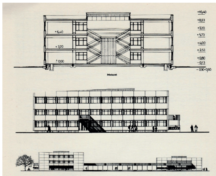
3. kép: A miskolci Vörösmarty Mihály Katolikus Általános Iskola és Óvoda metszete és homlokzatai Forrás: Kmetty Gyula [szerk.]: Északterv Műszaki Tájékoztató 1978. Építésügyi Tájékoztatói Központ, Budapest 1979, 98.
